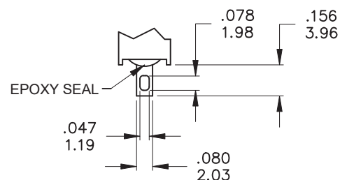
SOLDER LUG
